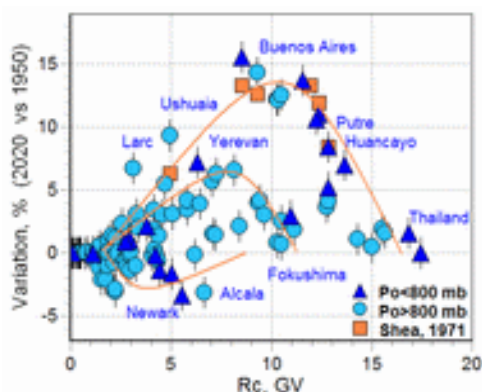
Рис. 3. Вековые вариации нейтронной компоненты станций космических лучей. Треугольники - горные станции.
