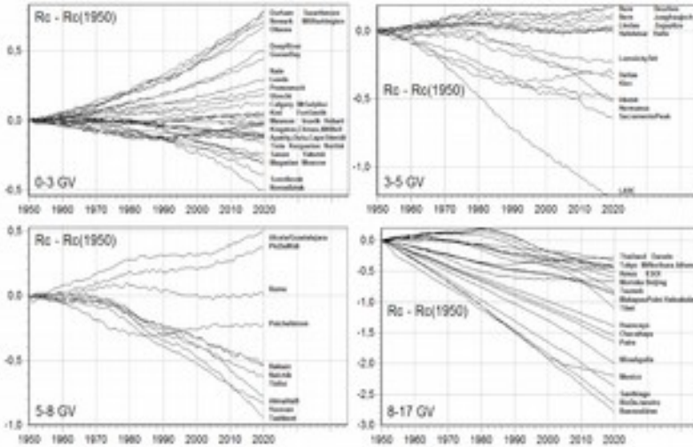
Рис. 2. Относительное изменение вертикальных жесткостей геомагнитного обрезания относительно эпохи 1950.
