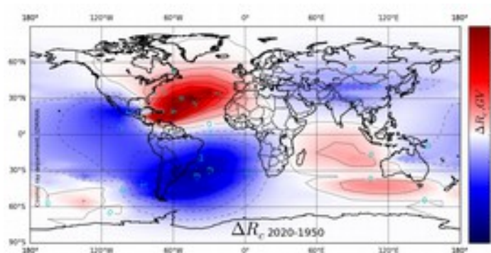
Рис. 1. Изменения планетарного распределения вертикальной жесткости геомагнитного обрезания относительно эпохи 1950. [Mag_Effect, 2016].
